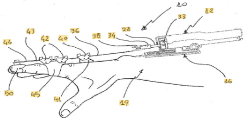
Fig 6.2. Vista frontal
